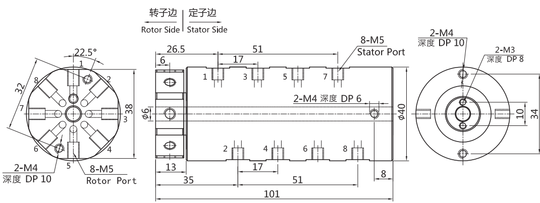
3008004 (8进8出, 4~6mm气管, 纯气动旋转接头) 尺寸图
