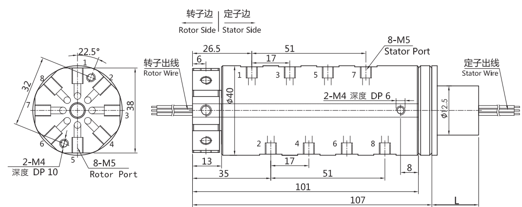
3008004 (8进8出, 4~6mm气管) +6~36路信号系列尺寸图 (适用于电磁阀与感应开关)
